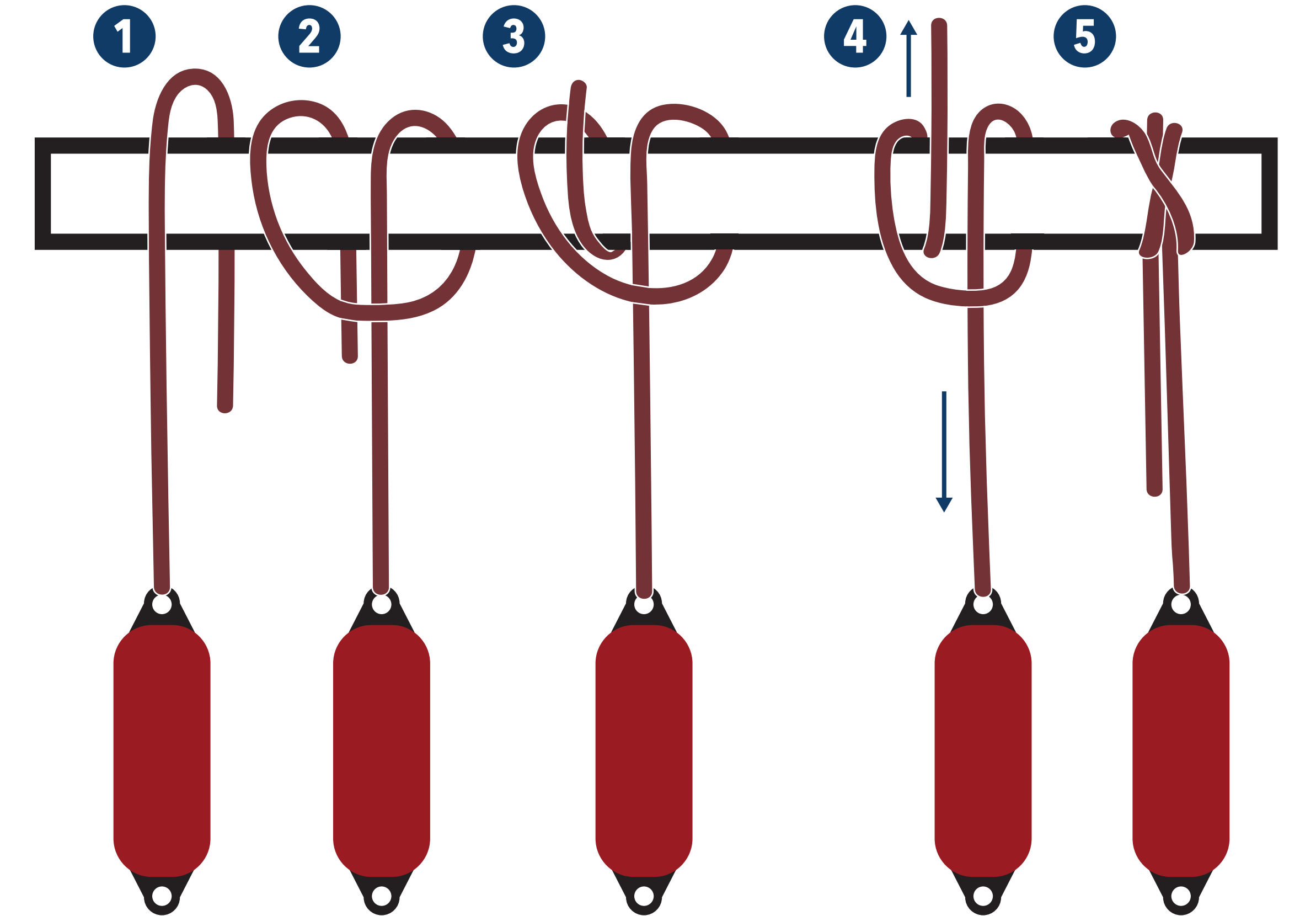
BALLESTRINQUE
